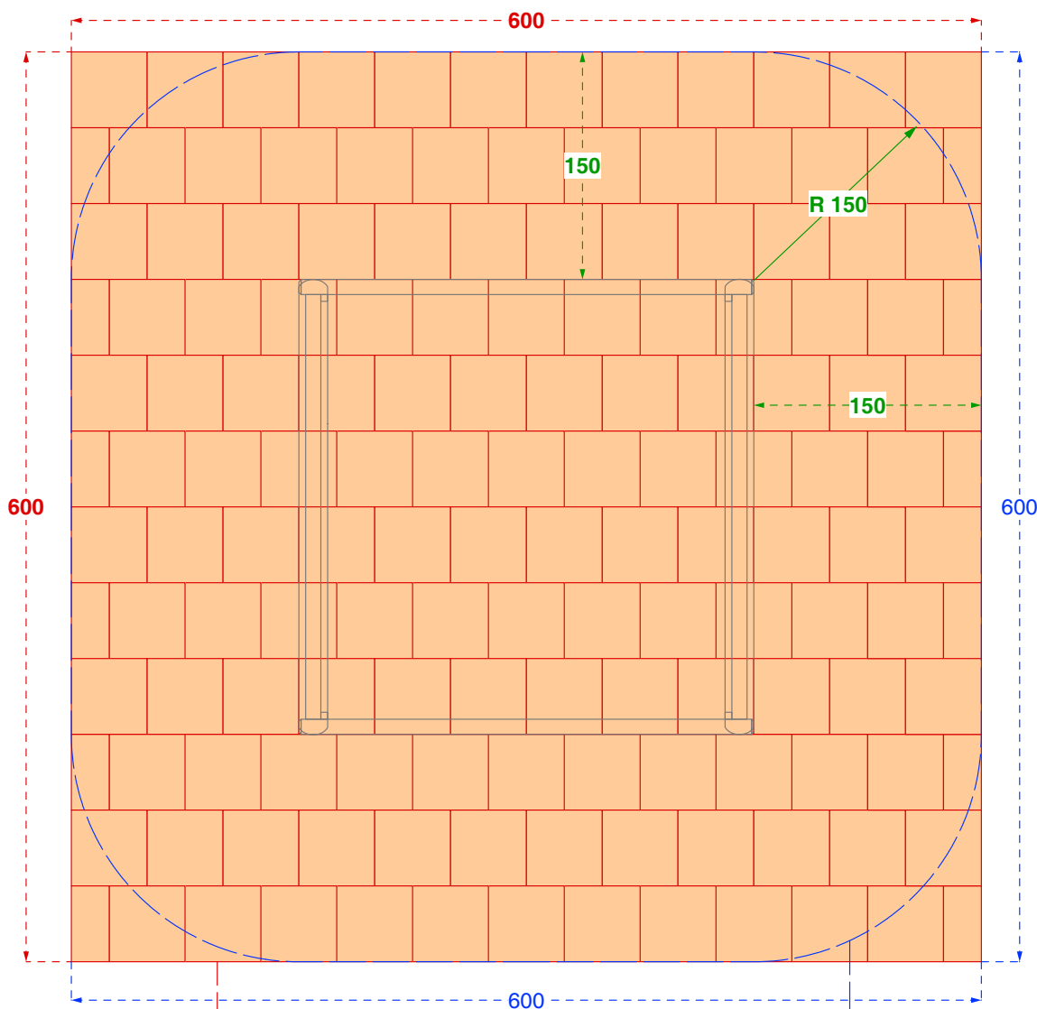
SPAZIO DI CADUTA / FALL SPACE
