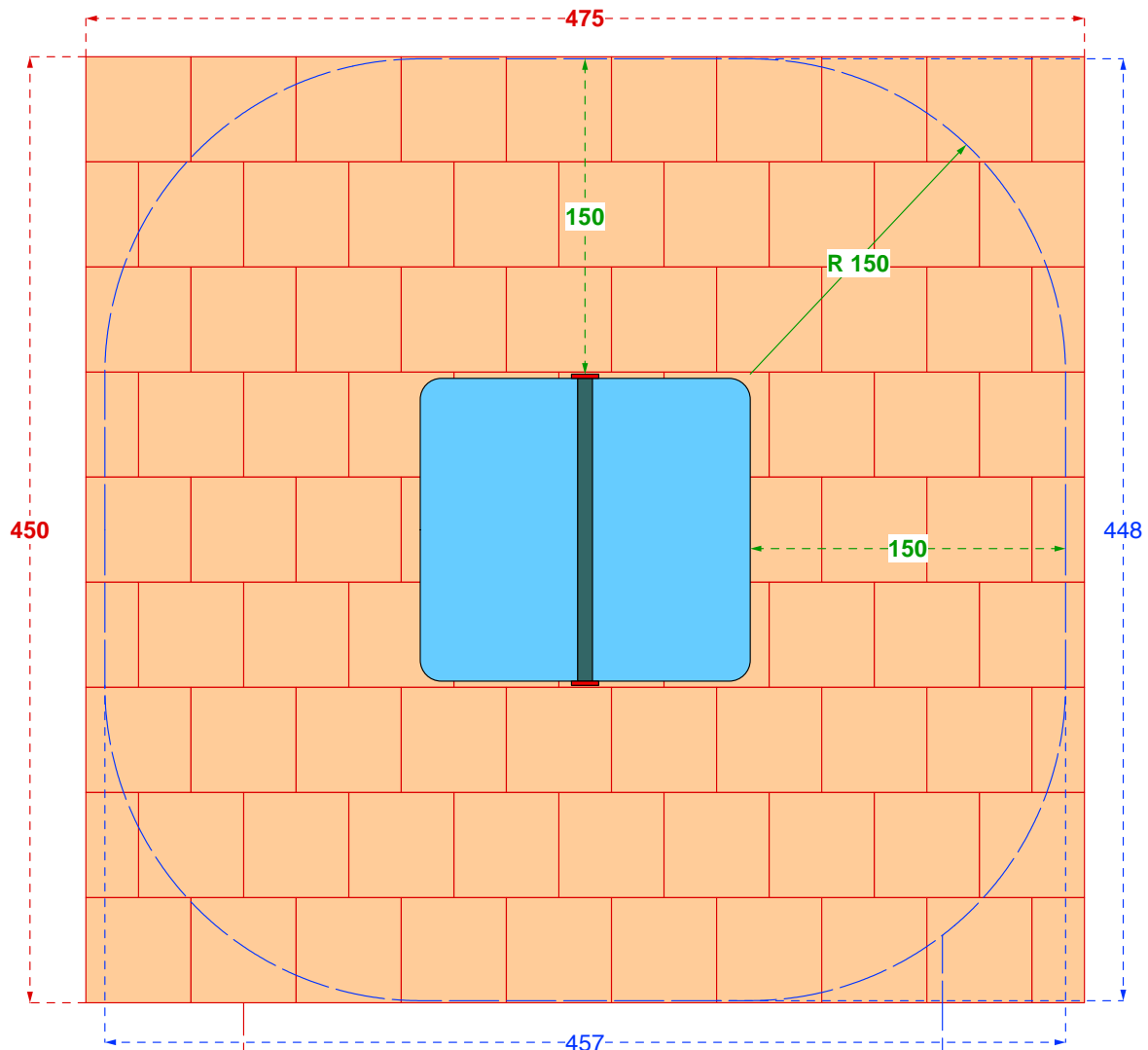
PAVIMENTAZIONE IN PIASTRE ELASTICHE / ELASTIC TILES PAVEMENT
